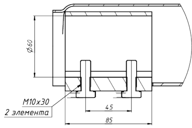
Вид - А
